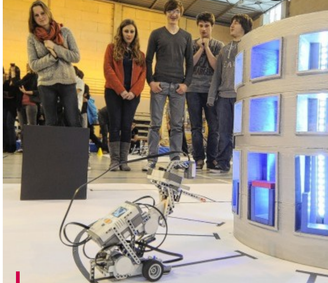
Dans l'épreuve de télémanipulation, le robot devait retirer des composants pour les acheminer et les déposer dans une zone de maintenance.
