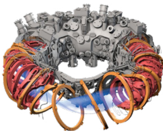
Fig. 2 : Schéma de la configuration magnétique d'un stellarator (ici W7-X). Les bobines externes (en rouge) produisent le champ magnétique total. Une surface magnétique est représentée en bleu.
