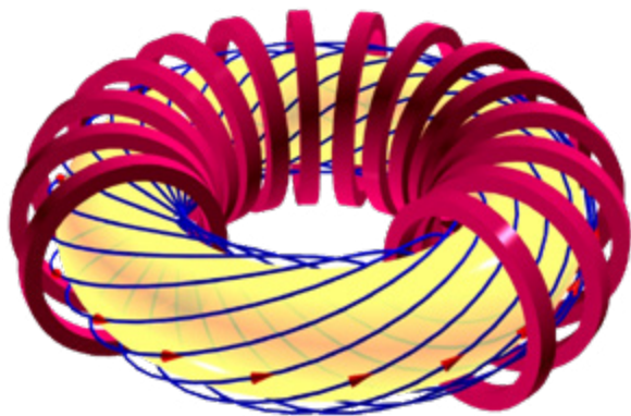
Fig. 1 : Schéma de la configuration magnétique d'un tokamak. Les bobines externes produisant le champ magnétique toroïdal sont représentées en rouge. La circulation d'un courant dans le plasma produit une composante additionnelle dans la direction poléoïdale et la trajectoire des lignes de champ (en bleu) s'enroule en hélice sur une surface (en jaune).
