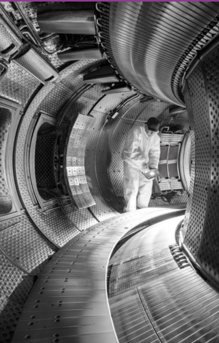
Fig. 3 : Intérieur du tokamak WEST (CEA-IRFM - France)
