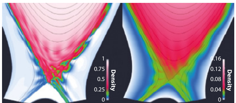
Fig. 2 : Perturbation de densité (à gauche) et de température (à droite) dans le plan polaire au moment du maximum de perturbation magnétique d'un ELM (code JOREK).
