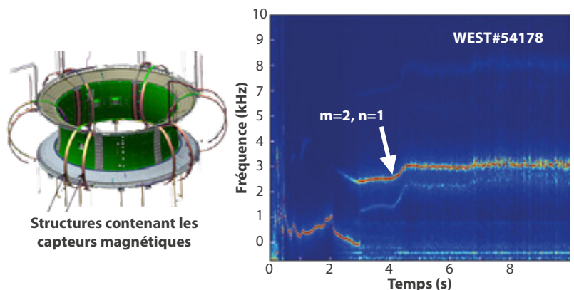
Fig. 1 : A gauche : position des capteurs de champ magnétique dans l'enceinte à vide de WEST. A droite : spectrogramme d'un capteur magnétique montrant l'évolution temporelle de la fréquence d'une perturbation magnétique se développant sur la surface rationnelle ( m=2 , n=1 ). L'amplitude de la perturbation est 10^5 fois plus faible que celle du champ magnétique principal.
