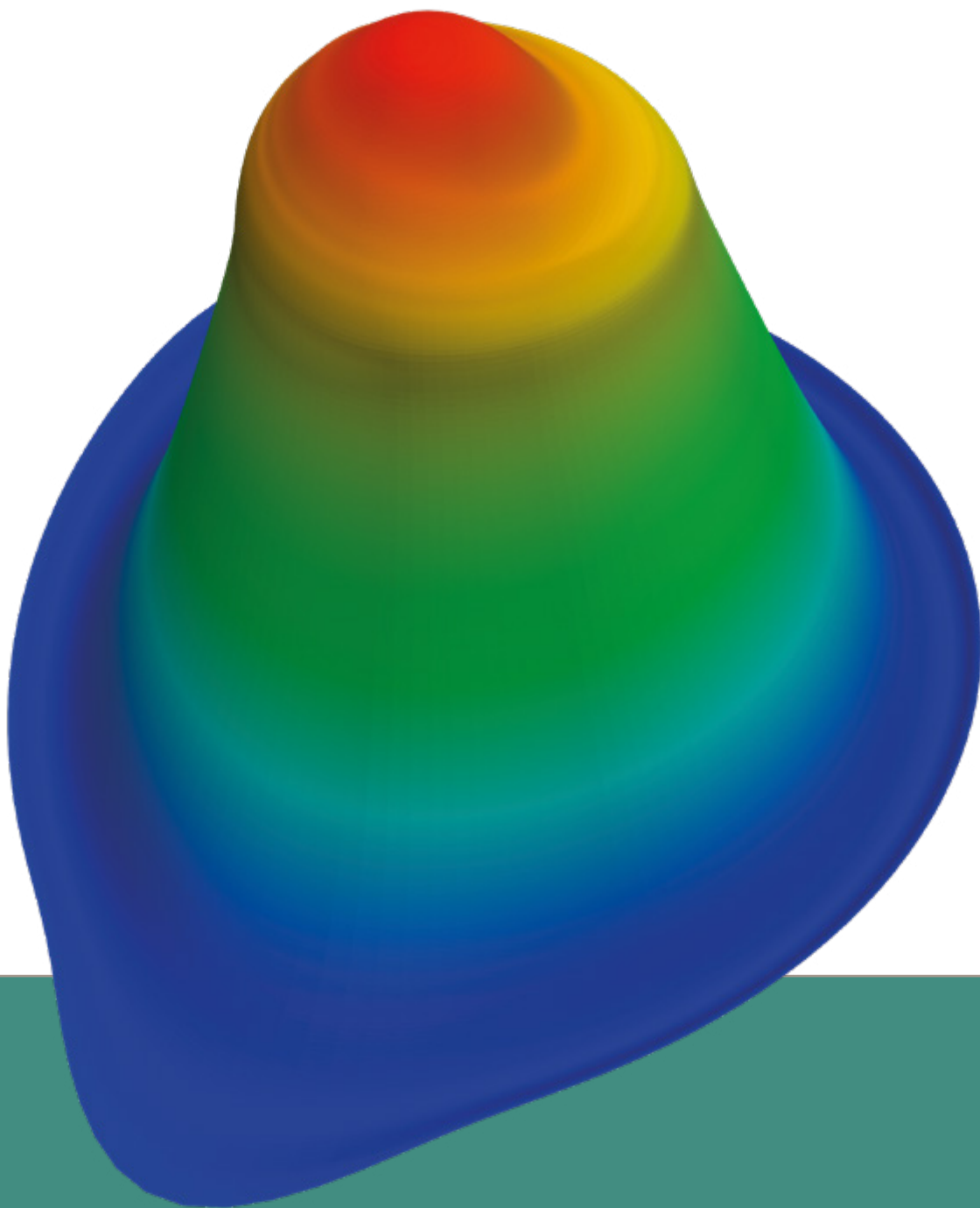
Fig. 3 : Température lors d'un crash de dent-de-scie dans WEST (visualisation d'une coupe poloïdale d'une simulation avec le code XTOR). On voit comment le cœur du plasma est déplacé vers l'extérieur. La surface de résonance de l'instabilité se situe approximativement à l'endroit où la température commence à décroître fortement.
