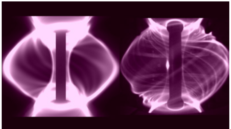
Fig. 1 : Images de caméra rapide et de simulations pour le tokamak MAST [2]. A gauche : image de caméra visible et rapide d'un ELM sur MAST. A droite : simulation avec le code JOEREK [3].
