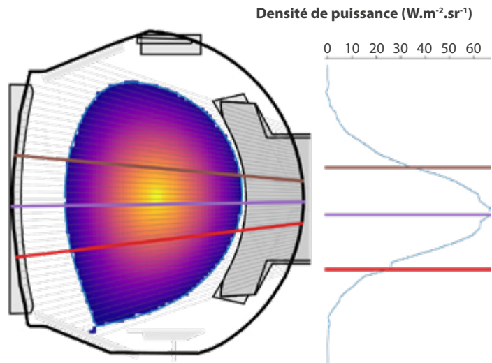
Fig. 4 : Carte 2D d'intensité du rayonnement X-mou (fort au centre, faible au bord du plasma) dans une section poloidale de WEST et surimpression des lignes de visées (en gris) du diagnostic associé, dont trois voies sont mises en avant. (droite) Signal associé.
