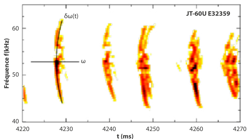
Fig. 1 : spectrogramme des fluctuations magnétiques représentant la fréquence d'un mode d'Alfvén en fonction du temps pour une décharge typique du tokamak japonais JT-60U. Le mode naît avec une fréquence \omega , qui est modifiée non linéairement vers le haut et vers le bas d'une quantité \delta\omega [3].
