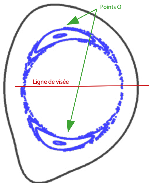
Fig. 1 : Température électronique mesurée en fonction du temps le long d'une ligne traversant le plasma (ligne rouge sur la figure de droite), en présence d'un îlot magnétique (en bleu sur la figure de droite), sur le tokamak WEST. La rotation naturelle du plasma fait que la présence de l'îlot se traduit par un aplatissement périodique du profil de température lors du passage des points O.
