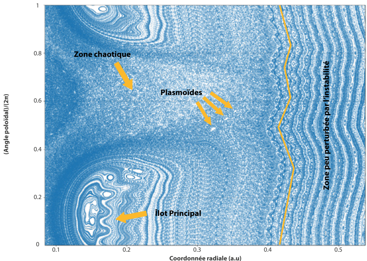
Fig. 2 : Coupe de Poincaré du champ magnétique, montrant l'îlot principal, des zones chaotiques, et de petits plasmoides le long de la zone de reconnexion, dans une simulation de dents-de-scie avec le code XTOR-2F [4].
