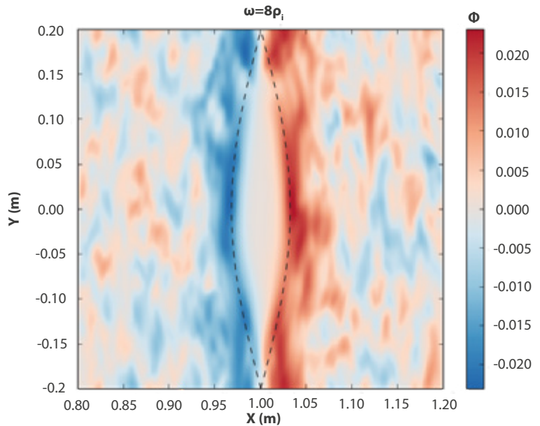
Fig. 1 : Amplitude des fluctuations turbulentes, en présence d'un îlot, issue de simulations numériques présentées dans [3]. Le transport parallèle aux lignes de champ magnétique correspond à la direction verticale, tandis que le transport perpendiculaire s'effectue de gauche à droite.
