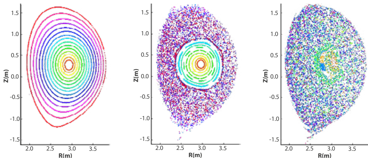
Fig. 3 : Résultats de simulation MHD avec le code JOREK [2] montrant des coupes de Poincaré du champ magnétique pendant la phase d'effondrement thermique d'une disruption (voir le texte pour des explications).
