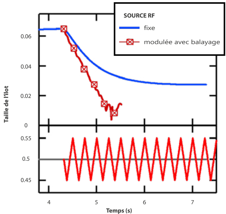
Fig. 2 : Simulation de contrôle d'un îlot magnétique par une source de courant avec le code XTOR [2] : la taille de l'îlot (en haut, en fraction du rayon du plasma) est réduite de moitié lorsqu'on lui applique une source de courant fixe (en bleu). Mais elle peut être réduite sous le seuil de détection lorsque le courant appliqué pour le contrôle est modulé au point O, tout en balayant radialement autour de sa position (en rouge). En bas, la position de la source de courant RF lors du balayage (l'îlot est à \rho_{RF}=0.5 ) [3].
