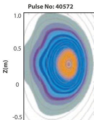
Fig. 1a : Section poloïdale du tokamak JET montrant le rayonnement X mou (couleurs) superposé aux surfaces magnétiques (traits gris). Ces dernières sont représentées à un instant où le plasma est stable, tandis que le rayonnement X est pris juste avant une disruption. La distortion des iso-contours du rayonnement est la marque d'un mode MHD global. (Figure extraite de G.T.A. Huysmans et al 1999 Nucl. Fusion 39 1489)
