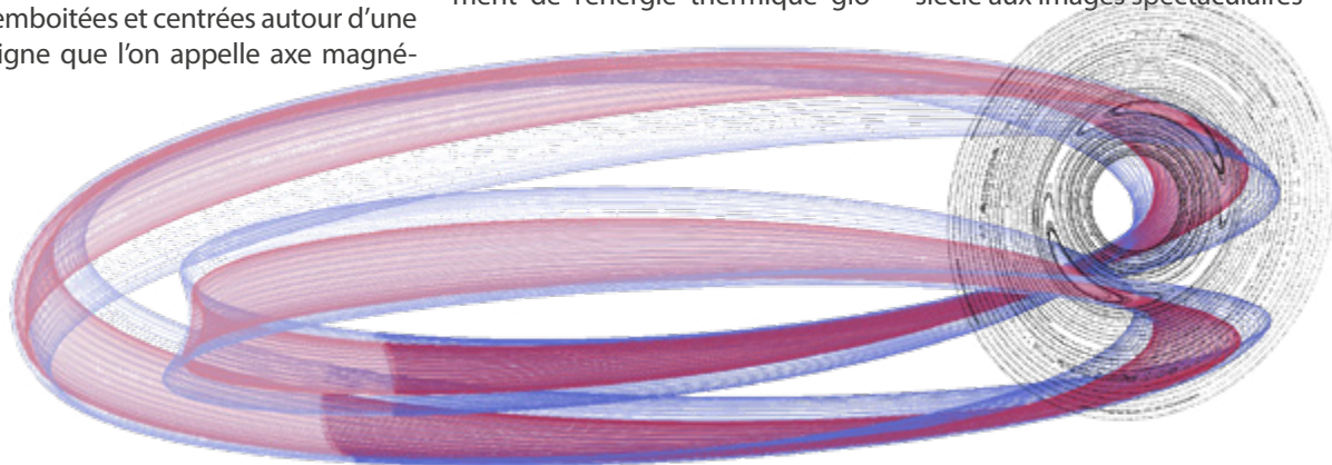
Fig. 2 : Surfaces magnétiques secondaires produites par un processus de reconnexion dans un tokamak . Les lignes de champ magnétique interceptent un plan poloïdal en formant la structure caractéristique d'un îlot magnétique .
