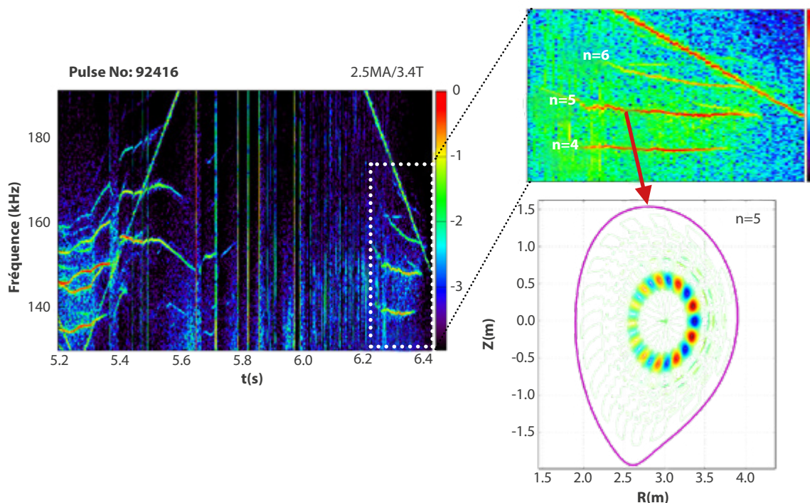
Fig. 2 : Spectrogramme mesuré dans un plasma de deutérium de JET. Les TAEs apparaissent comme des bandes colorées. (Droite, bas) Reconstruction numérique d'un des TAEs ( n=5 ) apparaissant sur le spectrogramme.
