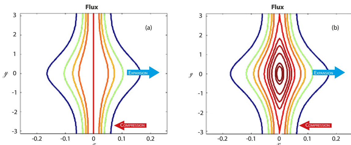
Fig. 1 : (a) Déformation des lignes de champ sur l'action d'un écoulement dans le cas d'un plasma idéal : pas de reconnexion. (b) Cas du plasma résistif : reconnexion et formation d'un îlot.
