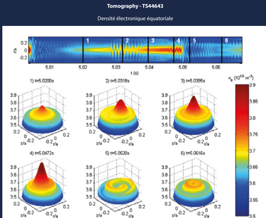
Fig. 3 : Reconstruction tomographique du profil de densité pendant une dent de scie.
