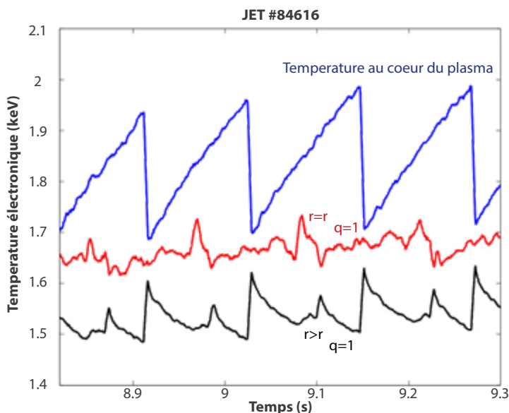
Fig. 1 : Traces temporelles de la température au cœur du plasma (bleu), à la surface de résonance de l'instabilité (rouge) et légèrement à l'extérieur de cette surface (noir), dans une décharge du tokamak européen JET.
