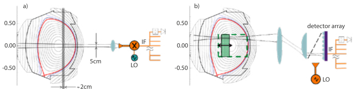
Fig. 2 : a) principe de la radiométrie 1D et b) principe de l'imagerie cyclotronique électronique
